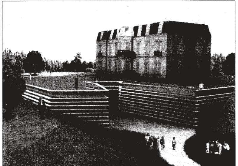
Fotomontaje del edificio semienterrado que se añadirá al Palacio de Aiete en su reconversión como centro cultural.
